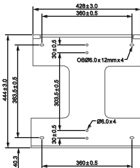
Fig. 4-1 - 1 Suspension murale pour onduleur photovoltaïque ES5500
