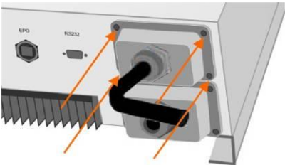
Fig. 8-1-3 – 5 Fixation du recouvrement
