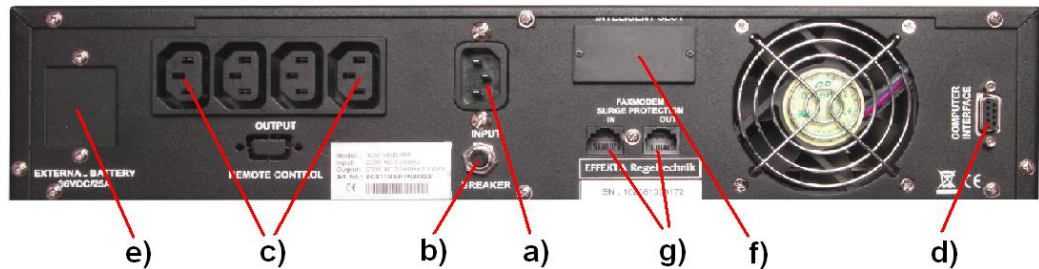
Abb. 3: Rückwand- Ansicht MKD700/1000
