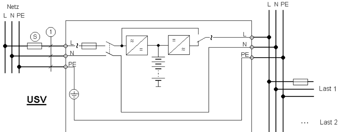
Abb. 4: Anschluss der USV
